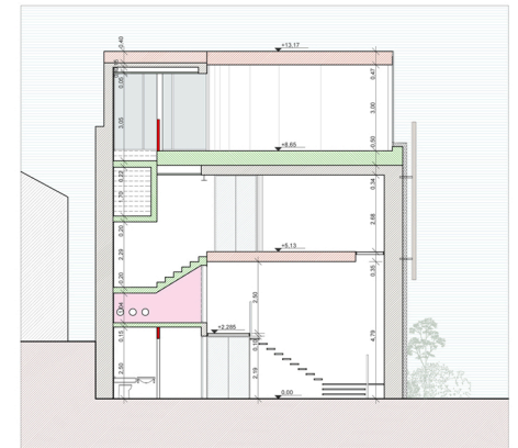
SEZIONE C-C''
