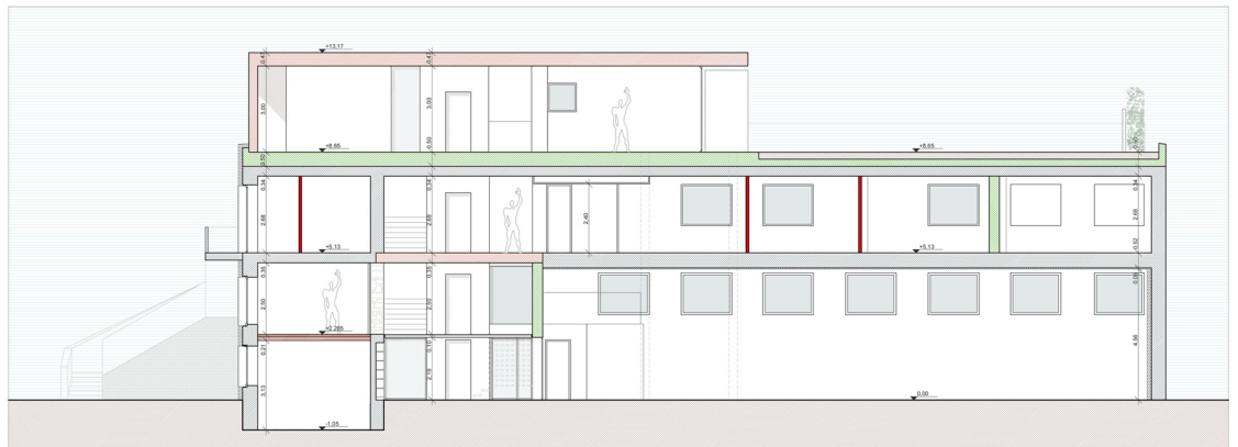
SEZIONE E-E
