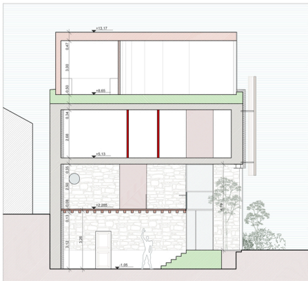
SEZIONE A-A'
