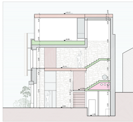
SEZIONE B-B
