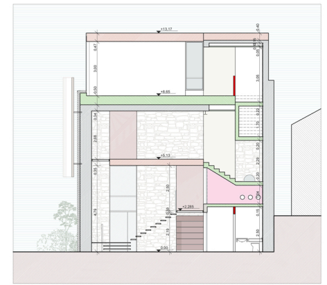
SEZIONE C-C
